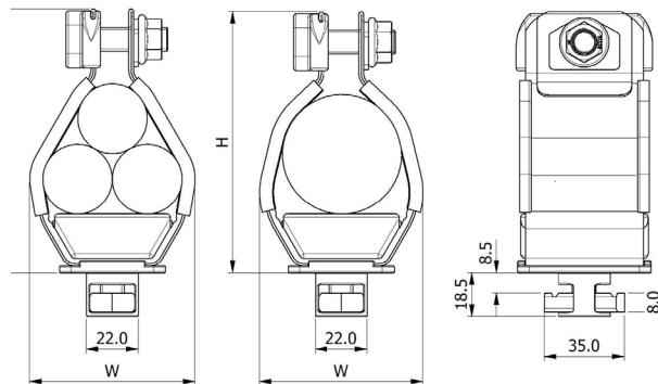
EINFACHER, FIXIERTER DREHFUSS: VRT+00 BIS VRT+12
