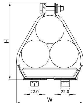
DOPPELTER, FIXIERTER DREHFUSS: VRT+13 BIS VRT+20
